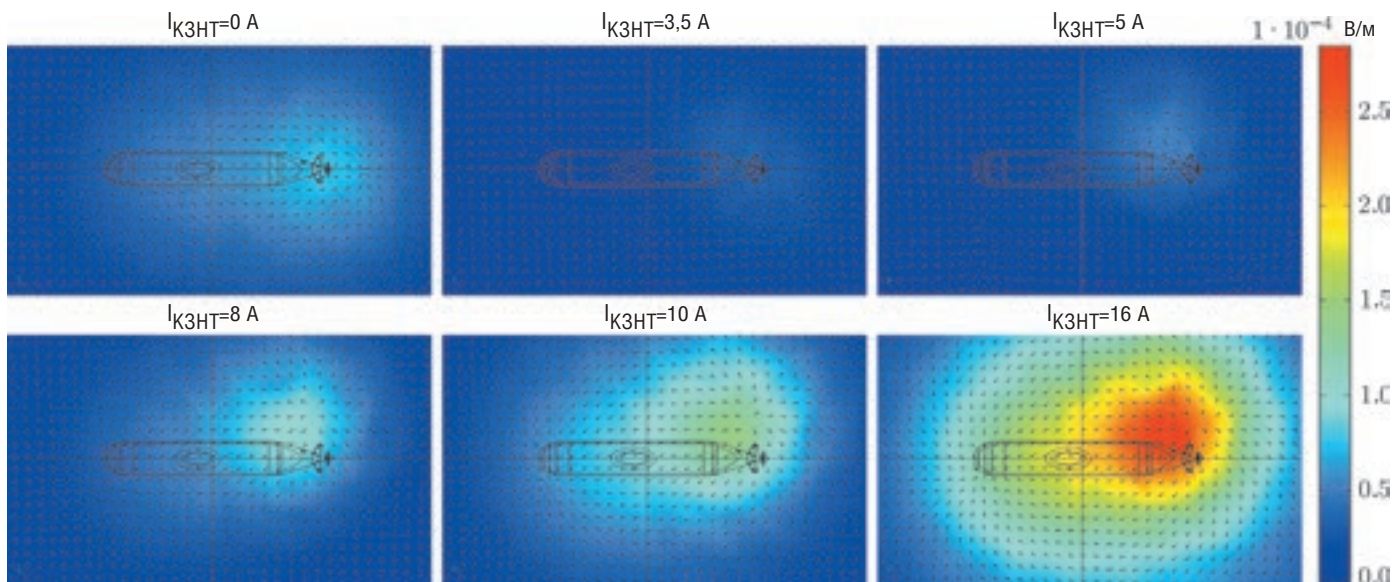
Рис. 4. Плоскости сигнатур электрического поля на глубине 20 метров ниже уровня киля для различных токов, наложенных системой КЗНТ. Сигнатура четко видна, когда система КЗНТ отключена (сверху слева) и достигает оптимального значения при силе тока 3,5 А (сверху посередине). С другой стороны, чрезмерная защита приводит к усилению сигнатуры ЭППЛ (ток КЗНТ равен 16 А, снизу справа).
