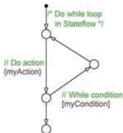
Рис. 2. Шаблон проектирования цикла с условием продолжения (do-while) в Stateflow
