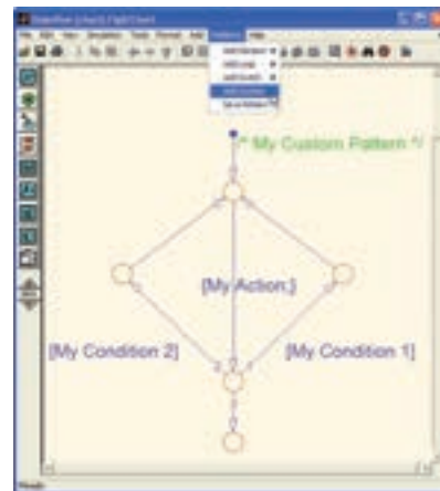
Рис. 8. Пользовательский шаблон моделирования, добавленный в Stateflow Design Pattern Wizard
