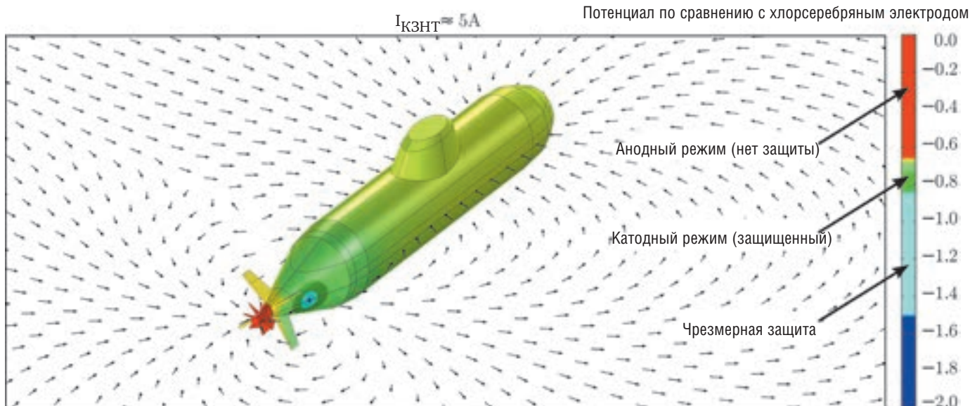
Рис. 2. Распределение потенциалов при наложении катодной защиты. Стрелки символизируют направления векторов напряженности электрического поля. В нормальных условиях работы для обеспечения катодного режима по всему корпусу ток КЗНТ должен быть незначительно выше (значение тока КЗНТ около 8 А). Палитра основана на немецкой морской инструкции VG 81259.
