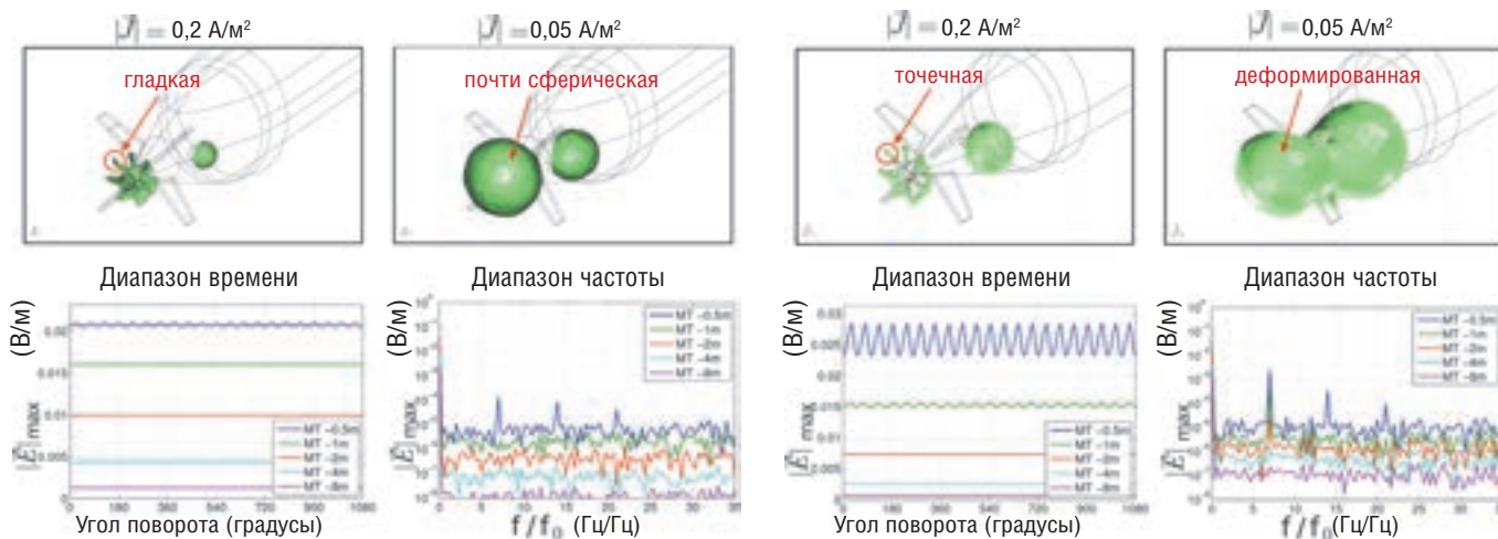
Рис. 3. Результаты симулирования модуляций ближнего поля, вызванных вращением гребного винта. Принятие упрощенных граничных условий Дирихле (слева) приводит к значительно большей модуляции, чем анализ граничных электрохимических реакций с использованием нелинейных кривых поляризации (справа).
