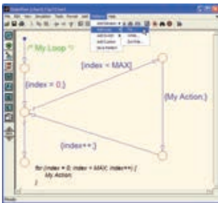
Рис. 7. Предварительно настроенный шаблон моделирования цикла for-while, добавленный в схему Stateflow
